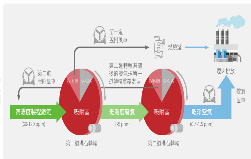
圖二、沸石濃縮雙轉輪系統示意圖
